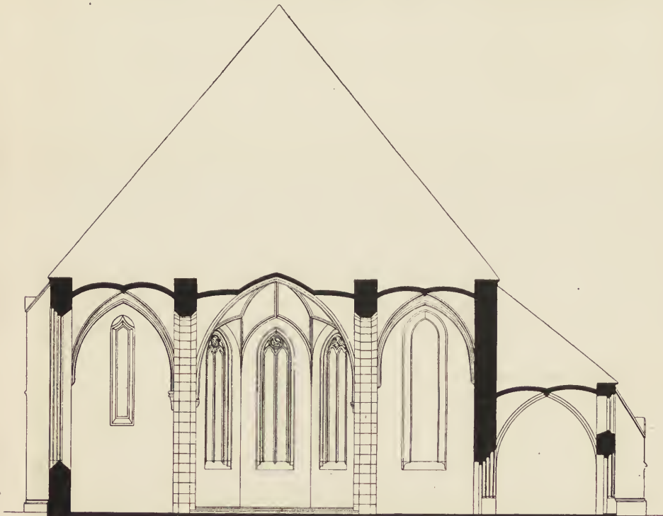
Fig. 28. St. Nicolaikirche. Querschnitt.
